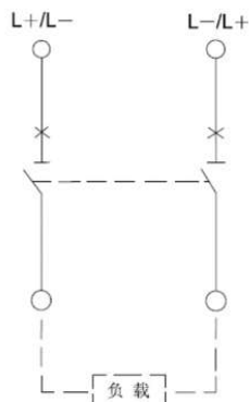
直流接线图：
